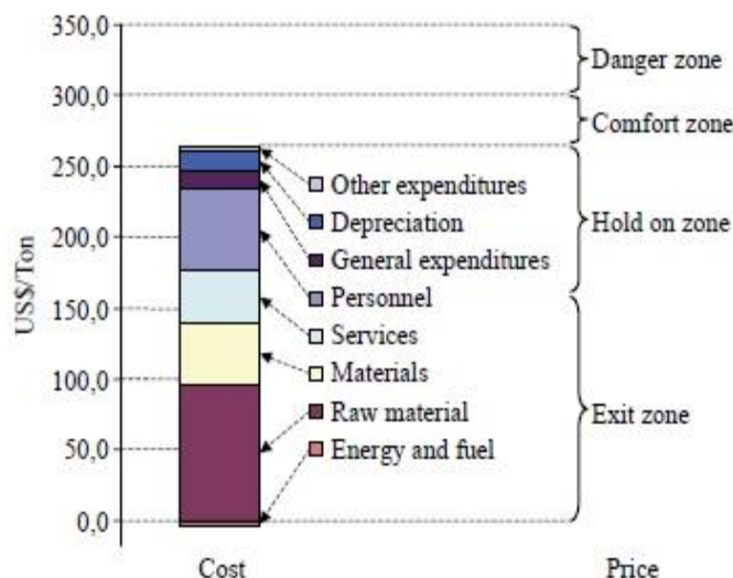
شکل (۲): نمودار هزینه محصول، استفاده از منابع و آستانه بهینه سازی
